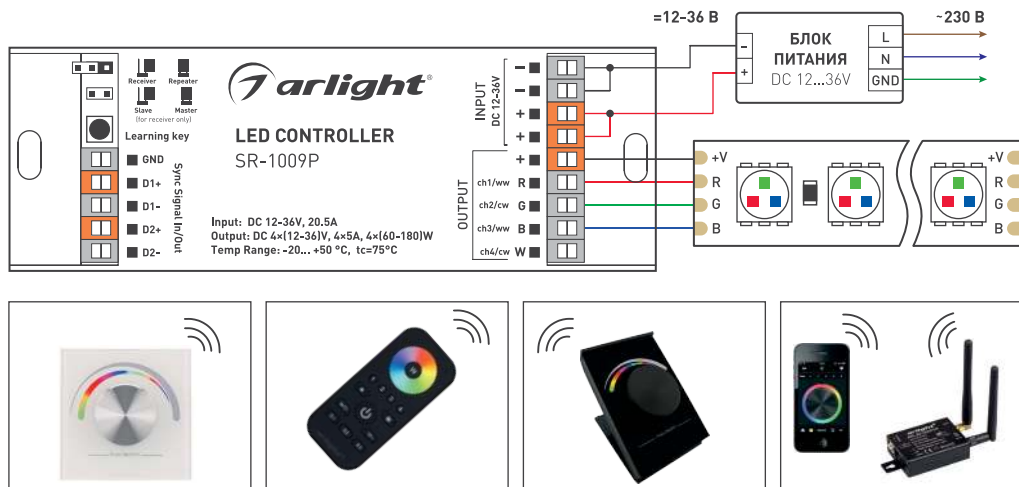
Рисунок 2. Схема подключения на примере контроллера SR-1009P.
