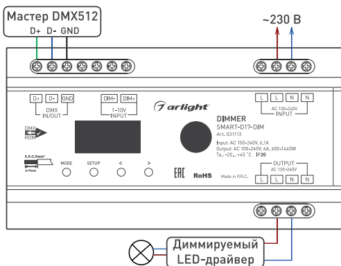
Рисунок 1. Схема подключения диммера SMART-D17-DIM в режиме DMX512
