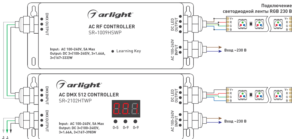
Рис.2. Использование контроллера SR-1009HSWP в качестве DMX мастер-контроллера на примере декодера SR-2102HTWP.
