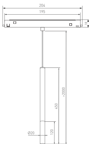
Рис. 1. Чертеж и габаритные размеры
