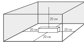
Рис. 3. Свободное пространство вокруг источника
