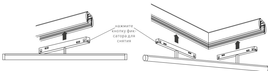
Рис. 2. Установка светильника
