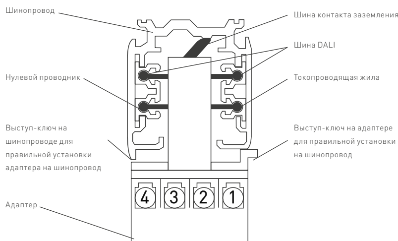
Рисунок 1. Подключение адаптера к шинпроводу
