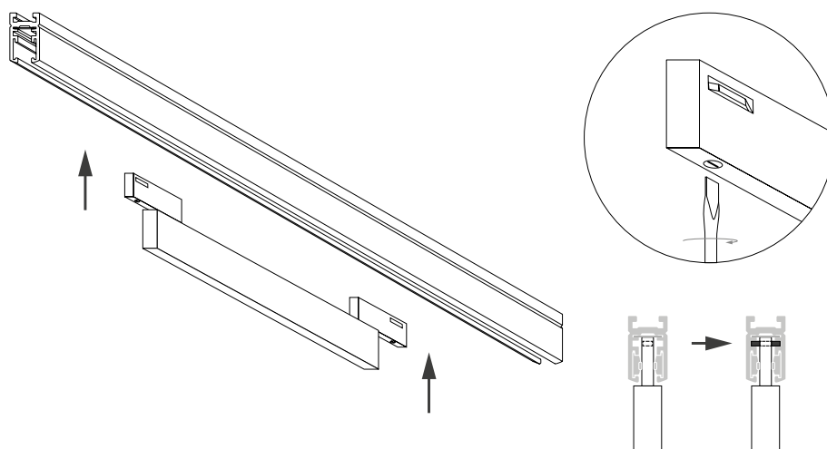
Рис. 2. Установка светильника
