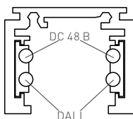
Рис. 3. Расположение контактов на шинопроводе
