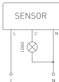
Рисунок 3. Схема подключения.
