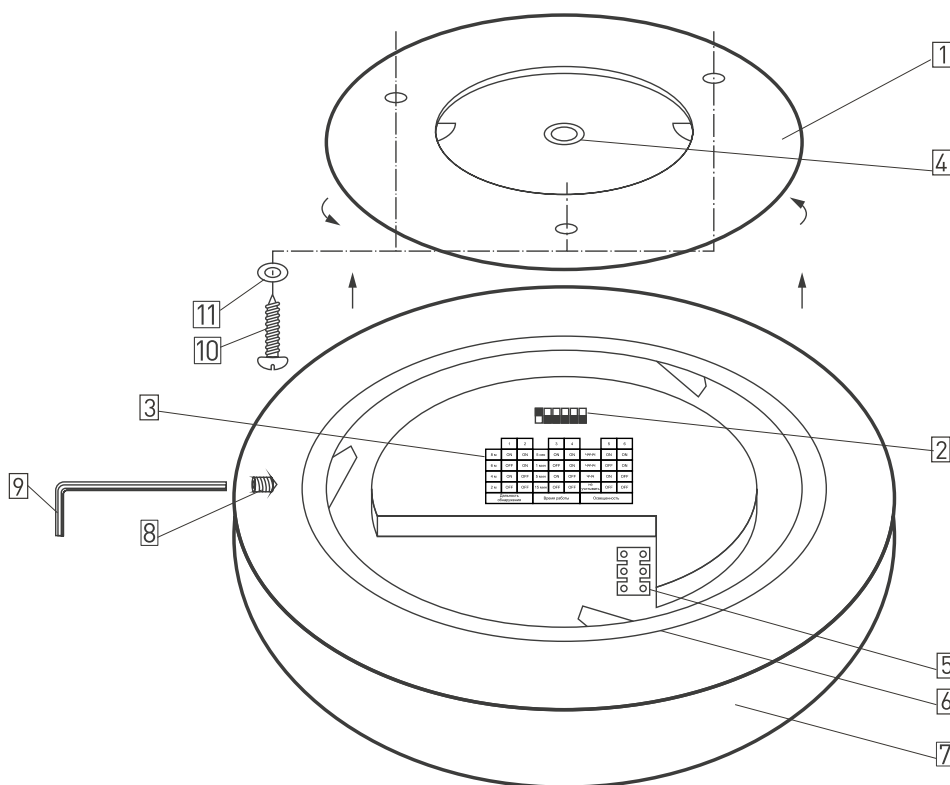
Рис. 3. Конструкция светильника
