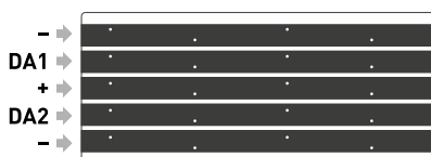
Расположение контактов на шинопровode
