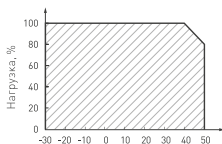
Рис. 2. Максимальная допустимая нагрузка, % от мощности источника
