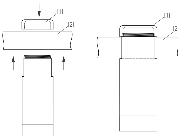
Рис. 2. Установка светильника
