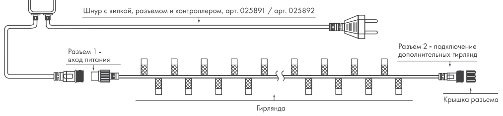
Рисунок 1. Схемы подключения.
