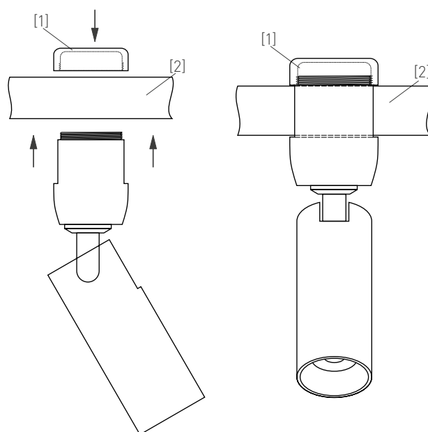
Рис. 2. Установка светильника
