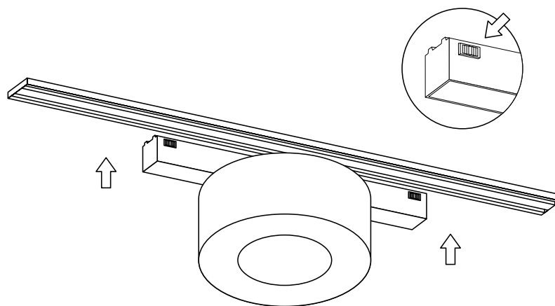
Рис. 2. Установка светильника
