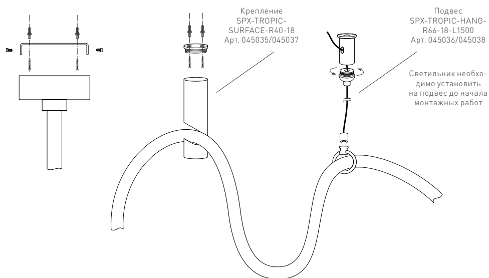
Рис. 2. Установка светильника
