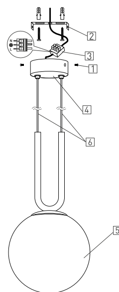
Рис. 2. Установка и подключение светильника
