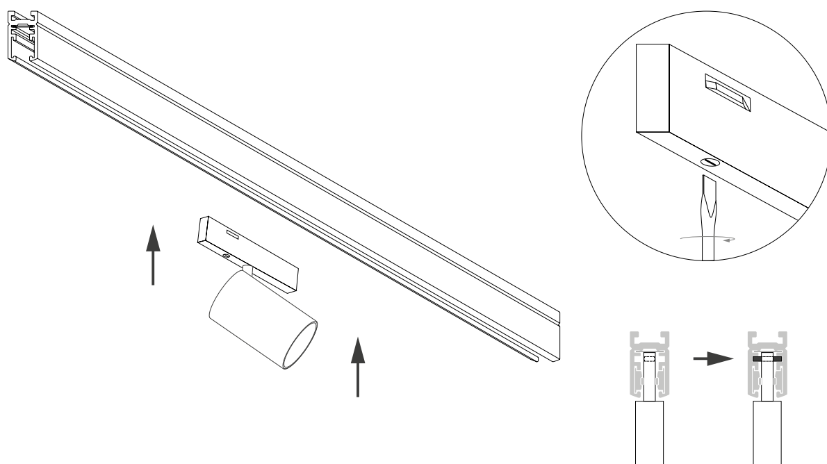
Рис. 2. Установка светильника
