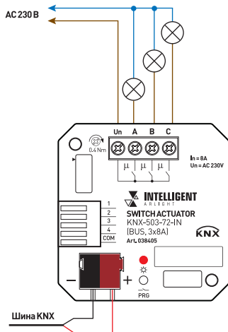
Рис. 1. Пример схемы подключения оборудования
