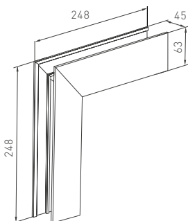
Коннектор угловой MAG-CON-4563-L90-EXT, для соединения типа внешний угол.
