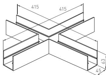
Коннектор крестовой MAG-CON-4563-X90, Х-образный коннектор.
