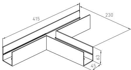
Коннектор тройной MAG-CON-4563-T90, Т-образный коннектор.
