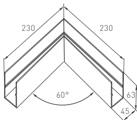
Коннектор угловой MAG-CON-4563-V60, L-образный коннектор 60°.
