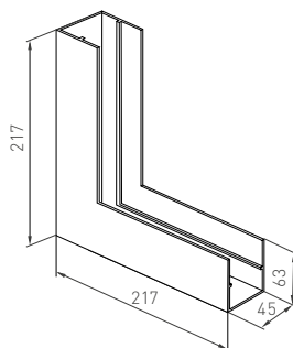
Коннектор угловой MAG-CON-4563-L90-INT, для соединения типа внутренний угол.
