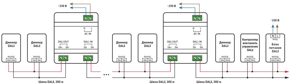
Рисунок 2. Схема подключения DALI-302-REP-DIN в качестве усилителя-ретранслятора сигнала DALI
