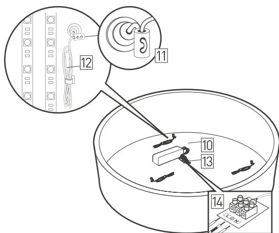
Рис. 2. Укладка кабеля
