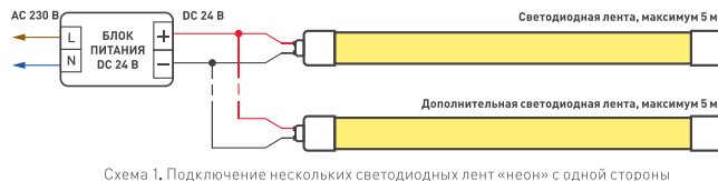
Схема 1. Подключение нескольких светодиодных лент «неон» с одной стороны
