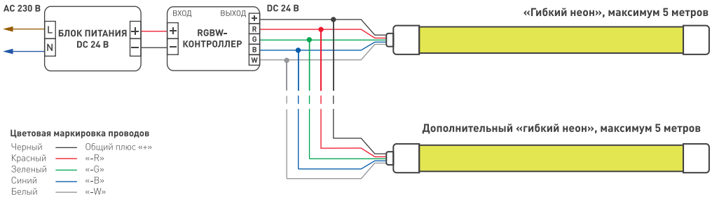
Схема 1. Подключение «гибкого неона» с использованием 4-канального RGBW-контроллера с возможностью изменения цвета свечения и яркости
