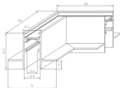
Коннектор угловой MAG-ORIENT-CON-2652-L90-FDW
