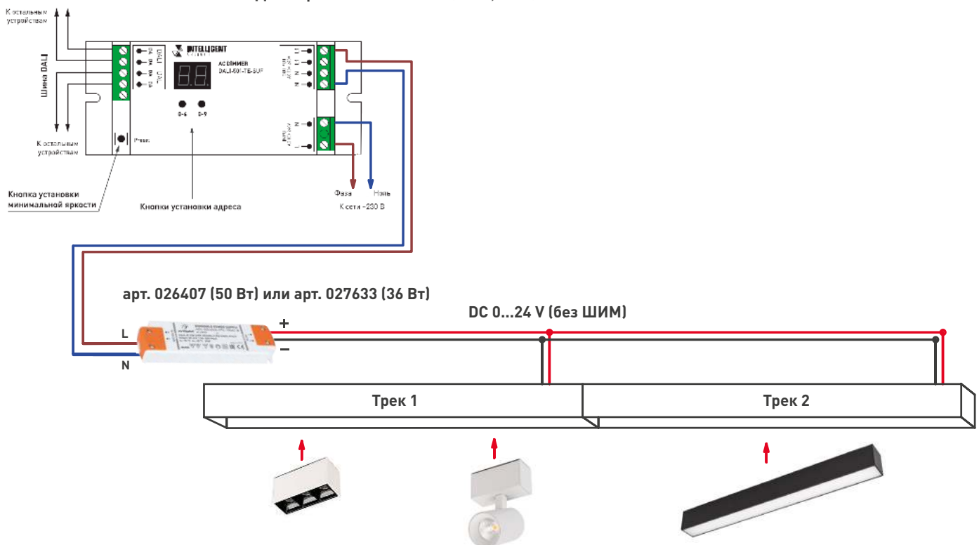
арт. 026403 INTELLIGENT ARLIGHT Диммер DALI-501-TE-SUF (230V, 2.2A)
