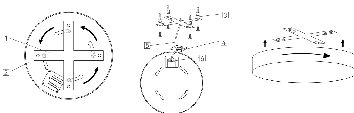
Рис. 2. Установка и подключение светильника
