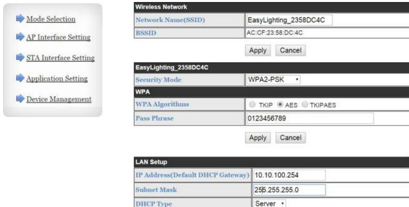
Рисунок 4. WEB-интерфейс конвертера.
