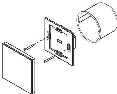
Рис. 2. Установка панели.
