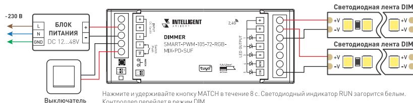
Рис. 1. Схемы подключения диммера SMART-PWM-105-72-RGB-MIX-PD-SUF
