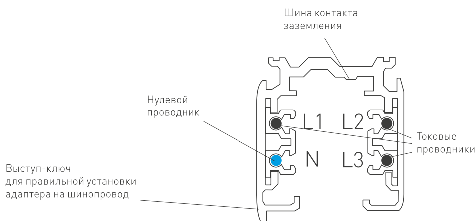
Рис. 1. Конструкция шинопровода
