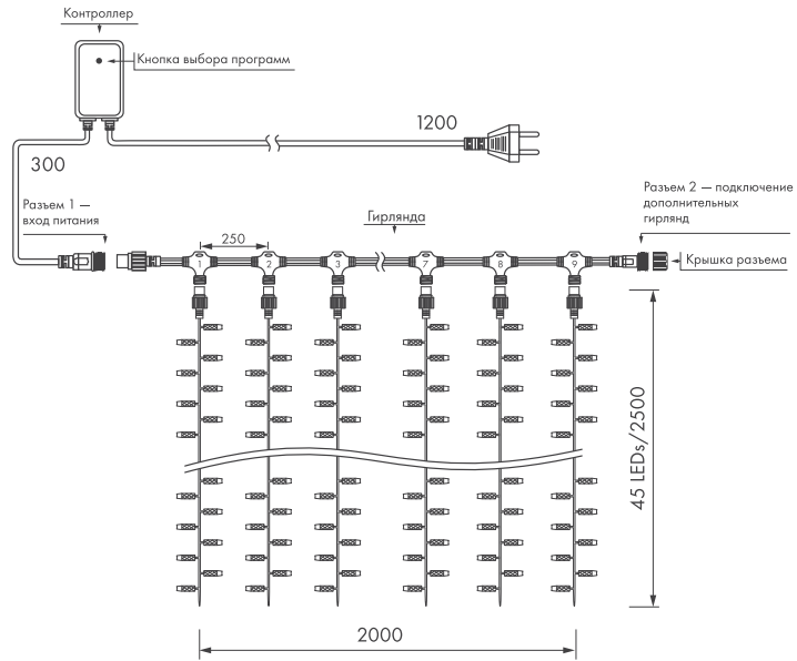
Рисунок 1. Схемы подключения
