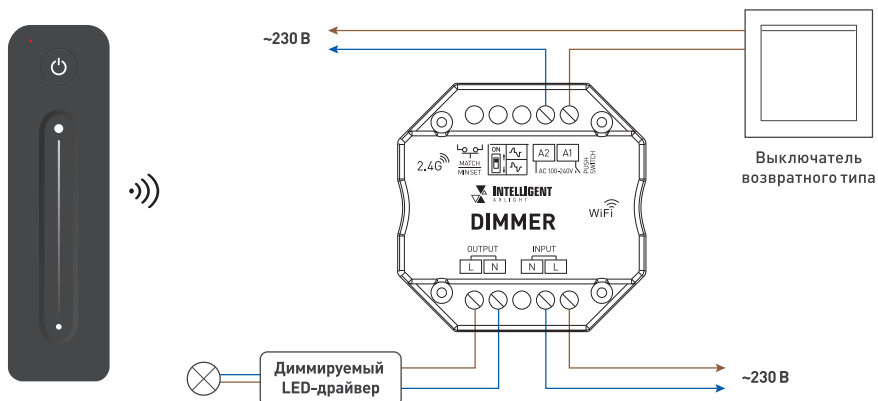
Рис. 1. Схема соединения оборудования
