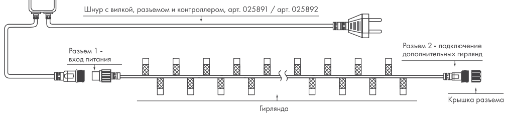
Рисунок 1. Схемы подключения.
