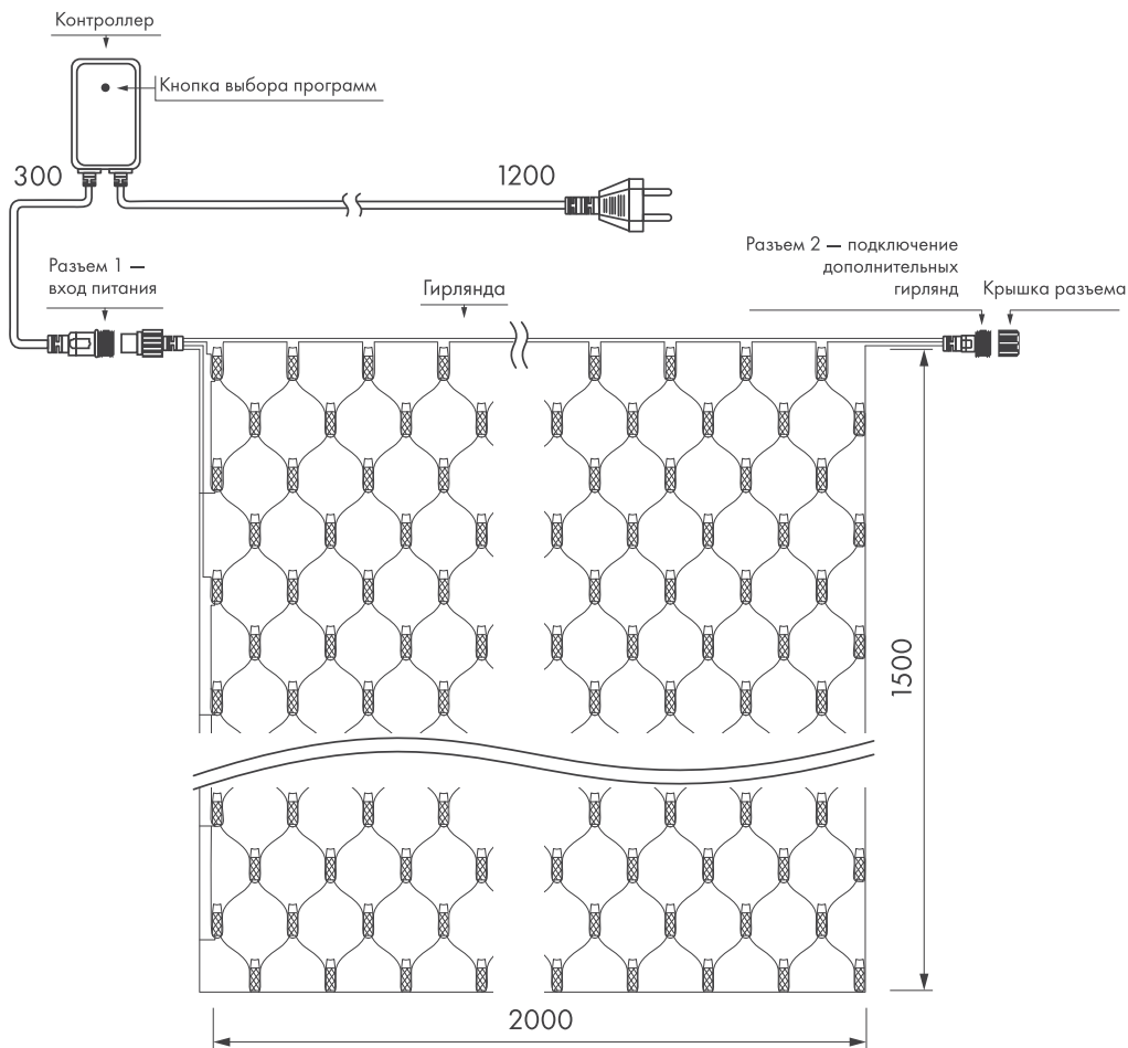
Рисунок 1. Схемы подключения.
