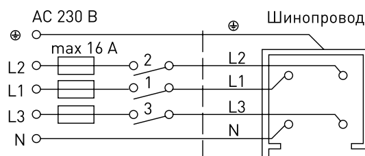
б) 3 фазы, 3 нагрузки, AC 230 В, 16 А, 3×3.7 кВА
