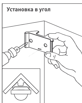
Рисунок 2. Варианты установки.
