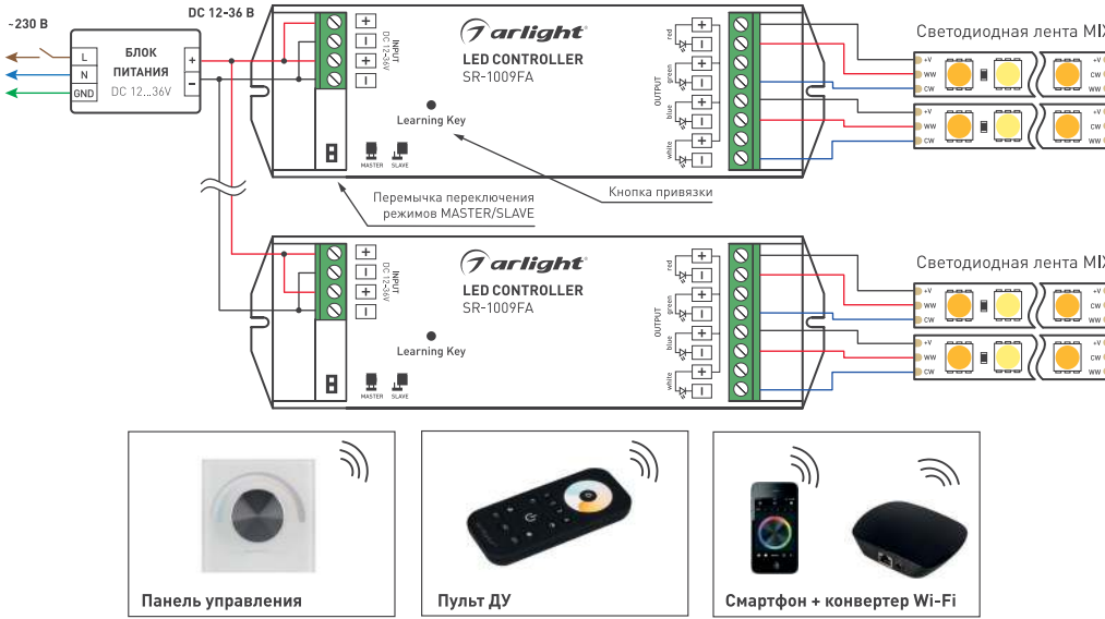
Рисунок 2. Схема подключения на примере контроллера SR-1009FA.
