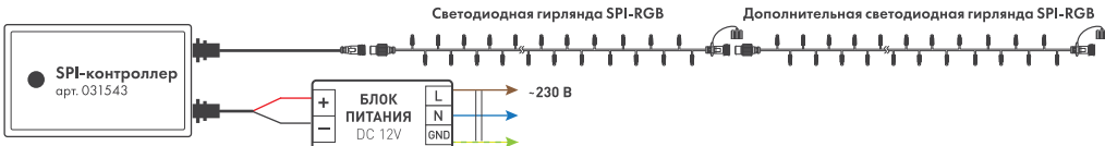
Рисунок 1. Подключение гирлянды с суммарной мощностью не более 80 Вт, при использовании SPI-контроллера арт. 031543 максимальное количество последовательно соединенных светодиодов/пикселей — 120 шт
