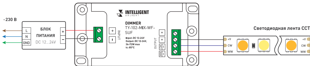
Рисунок 2. Пример схемы подключения диммера TY-102-MIX-SUF
