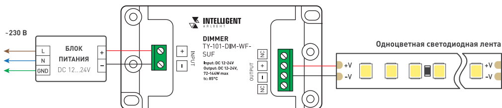
Рисунок 1. Пример схемы подключения диммера TY-101-DIM-WF-SUF
