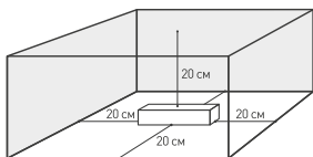
Рисунок 3. Свободное пространство вокруг источника
