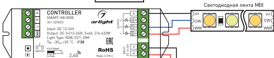
Рисунок 2. Подключение светодиодной ленты MIX
