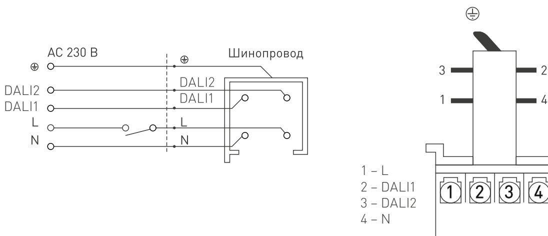
Рис. 2. Схема подключения
