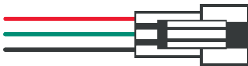
Рис. 3. Кабель для подключения лент SPI-B30 и SPI-SE-B30
