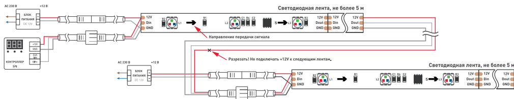
Рис. 2. Схема подключения ленты SPI-P-B30 с использованием SPI-контроллера с одним выходным портом и с использованием отдельных блоков питания
